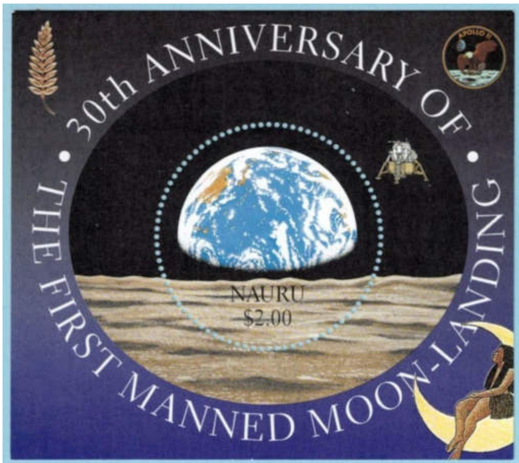
Die Erde als „Blauer Planet“
